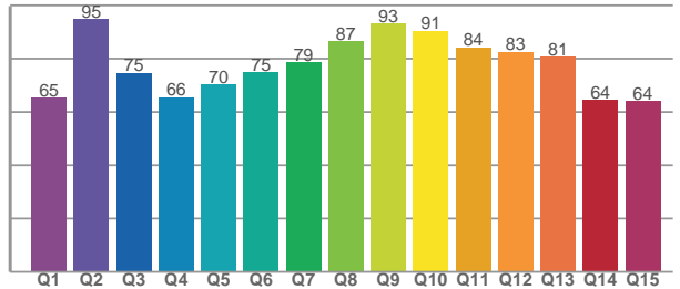
CQS: 75.6
