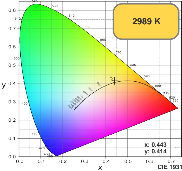
TM30: 78.8
