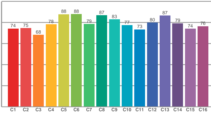
TM30: 78.8
