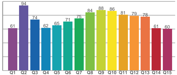
CQS: 72.4
