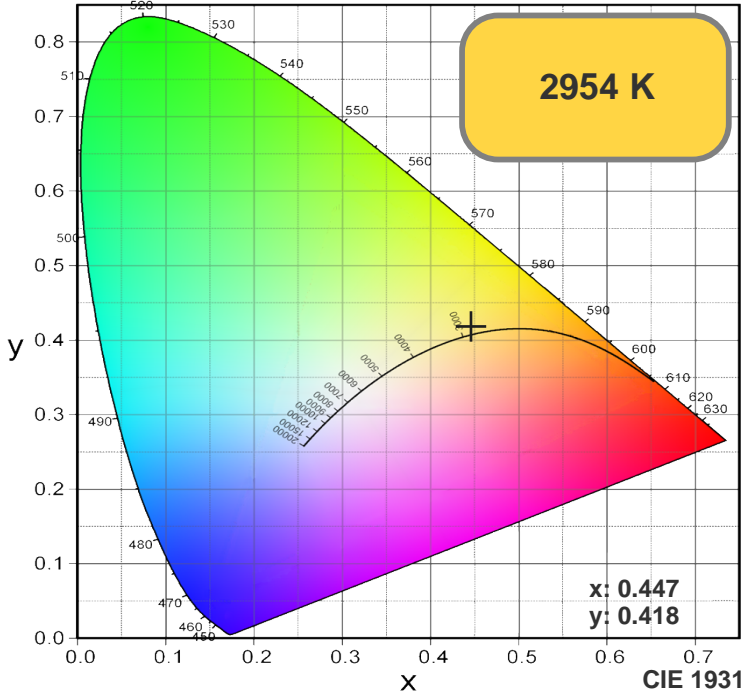
TM30: 78.5
