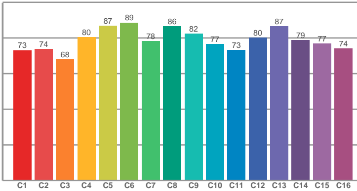
TM30: 78.5
