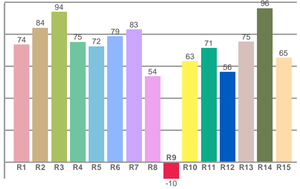
CQS: 72.4
