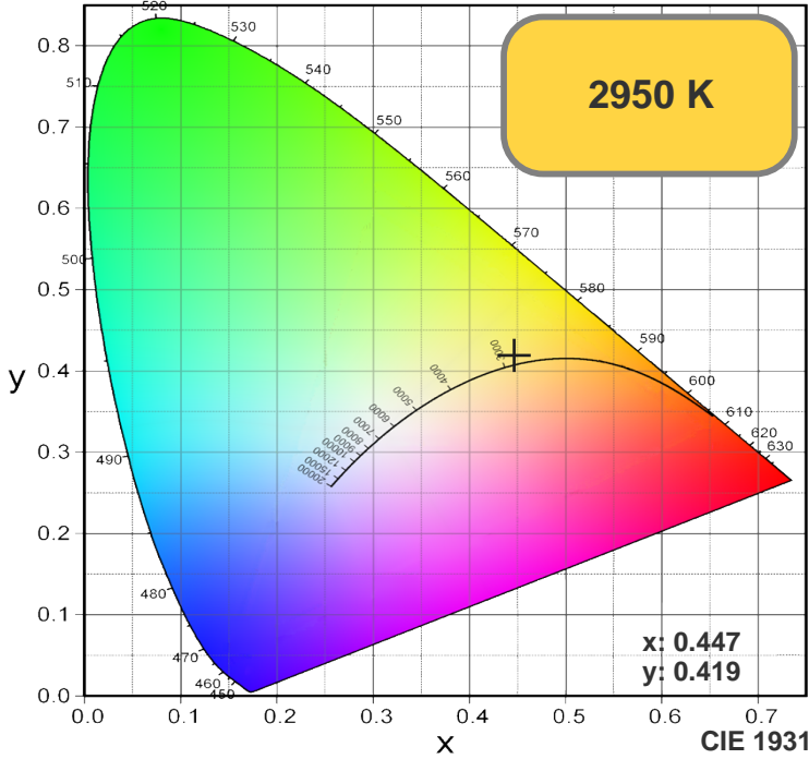
TM30: 78.6
