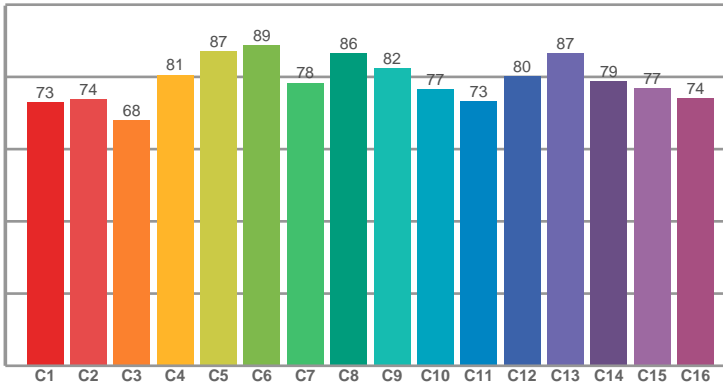
TM30: 78.6
